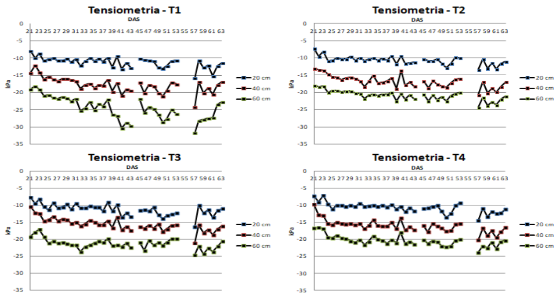
Figura 2. Valores de tensão nas profundidades 0,20, 0,40 e 0,60 m para os diferentes tratamentos.
