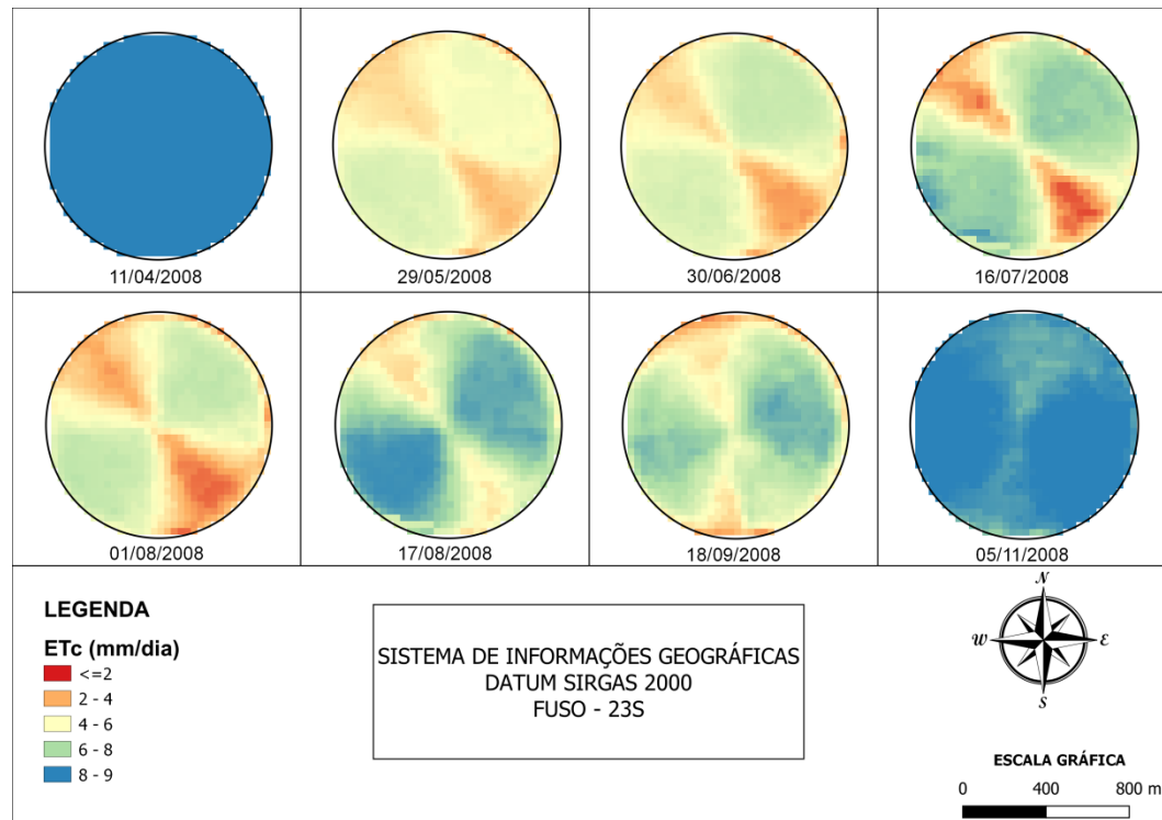
Figura 3. Evapotranspiração da cultura (ET c ), em mm d -1 , obtidos através do algoritmo SEBAL.
