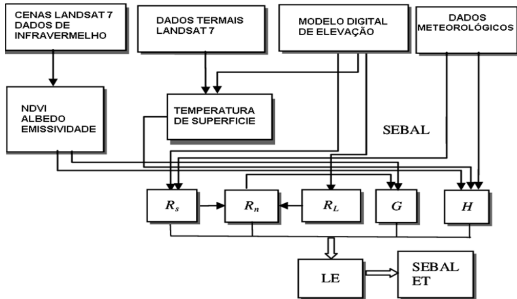
Figura 2. Rotina computacional do Modelo SEBAL; r_s é a radiação de onda curta incidente ( w m^{-2} ); r_n é o saldo de radiação ( w m^{-2} ); r_l é a radiação de onda longa emitida pela atmosfera ( w m^{-2} ); g é o fluxo de calor no solo ( w m^{-2} ); h representa o fluxo de calor sensível ( w m^{-2} ); le é o fluxo de calor latente ( w m^{-2} ).
