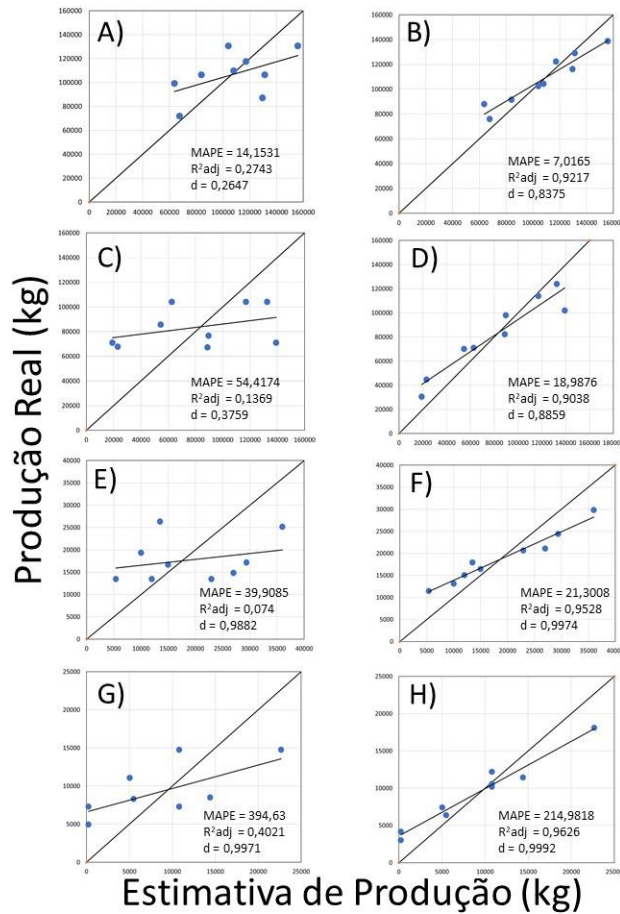
Figura 5. Comparação dos modelos de estimativa do milho para MS. A) Chapadão do Sul (KNN); B) Chapadão do Sul (RANDOM); C) Costa Rica (KNN); D) Costa Rica (RANDOM); E) Ponta Porã (KNN); F) Ponta Porã (RANDOM); G) Sidrolândia (KNN); e H) Sidrolândia (RANDOM).
