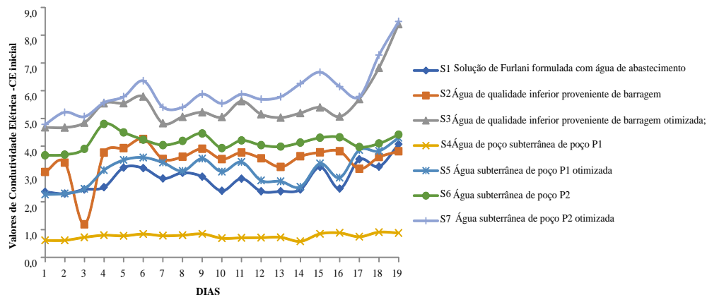
Figura 3. Variação da condutividade elétrica - CE ( \text{dS m}^{-1} ) das soluções nutritivas minerais S1; S2; S3; S4; S5; S6 e S7 (S1 = Solução de Furlani (água de abastecimento); S2 = Água de qualidade inferior proveniente de barragem; S3 = Água de qualidade inferior proveniente de barragem otimizada; S4 = Água subterrânea de poço P1; S5 = Água subterrânea de poço P1 otimizada; S6 = Água subterrânea de poço P2 e S7 = Água subterrânea de poço P2 otimizada) durante o período experimental com as cultivares da alface crespa.
