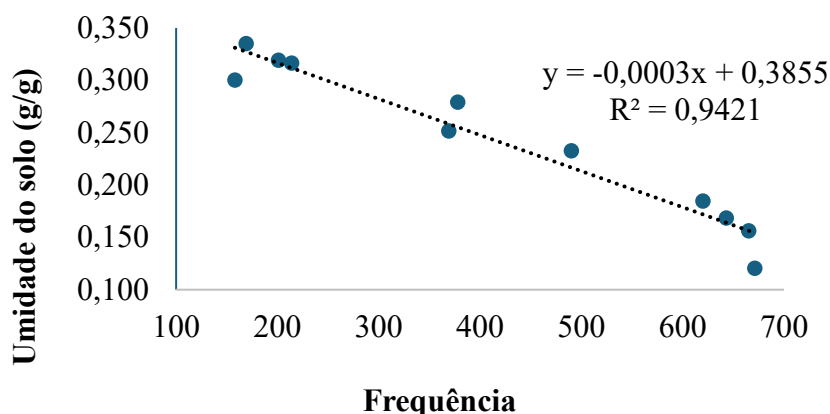
Figura 1. Gráfico de Calibração do Sensor de Umidade do Solo em Latossolo Vermelho.
